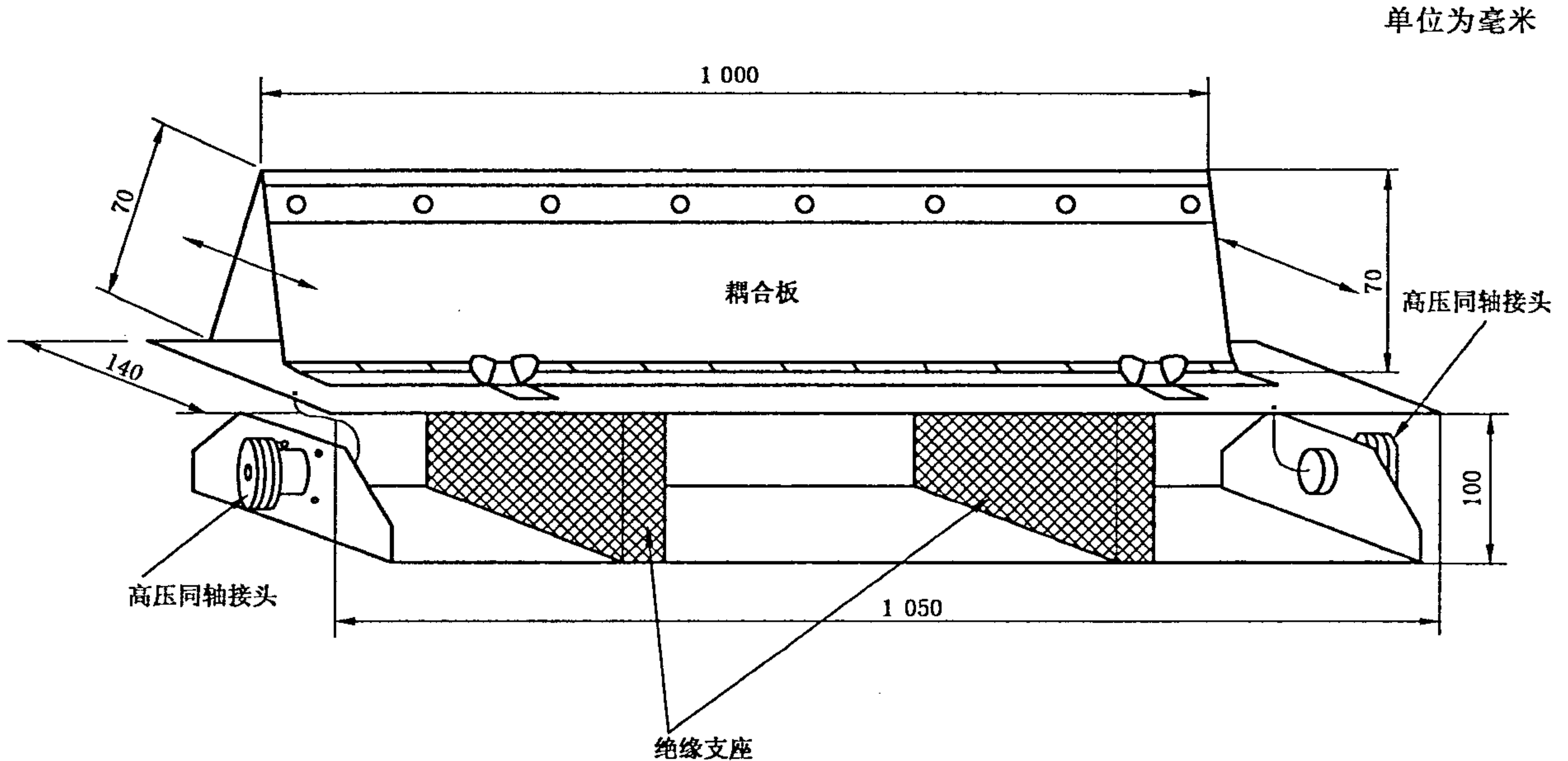
图 5 容性耦合夹的结构
