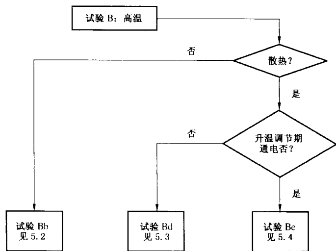
图 1 试验 B: 高温试验方框图
