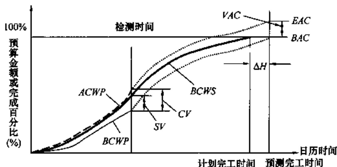
图 1 赢得值曲线
